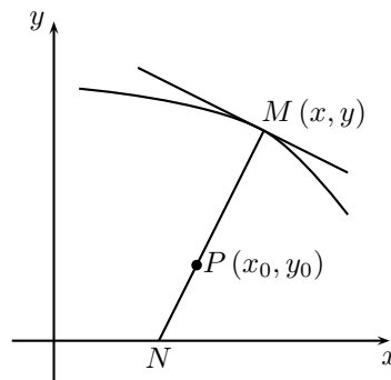
Figura 3.9: Problema geométrico.
