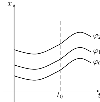
Figura 2.5: Solución única.
