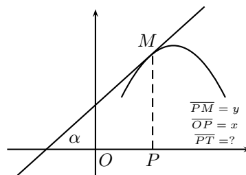
Figura 2.4: Problema geométrico.
