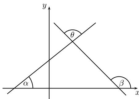
Figura 2.13: Rectas isogonales.
