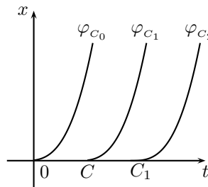
Figura 2.6: Soluciones múltiples.
