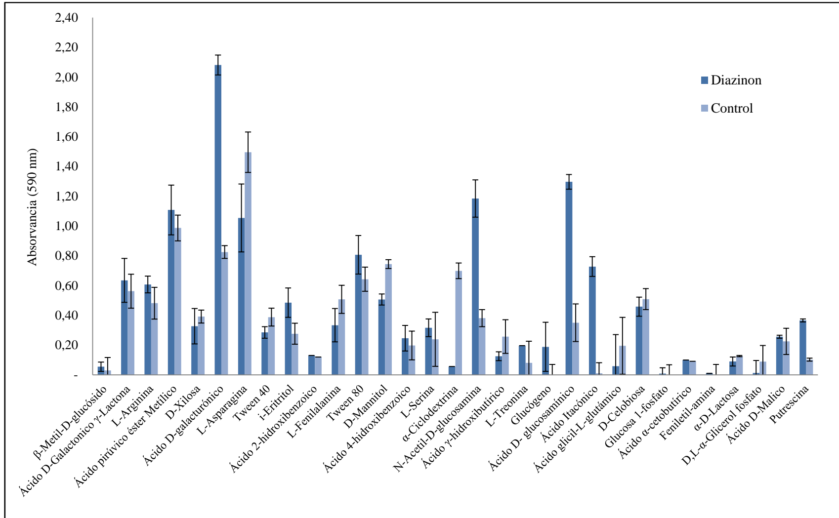
Figura 17. Perfil del nivel fisiológico de la comunidad microbiana (CLPP) al día 90 de evaluación.
