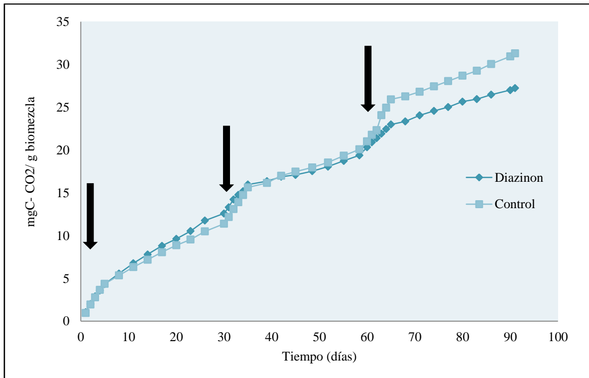
Figura 8. Efecto de 3 aplicaciones sucesivas de diazinón (40 mg ia kg -1 ) sobre la evolución del dióxido de carbono.
