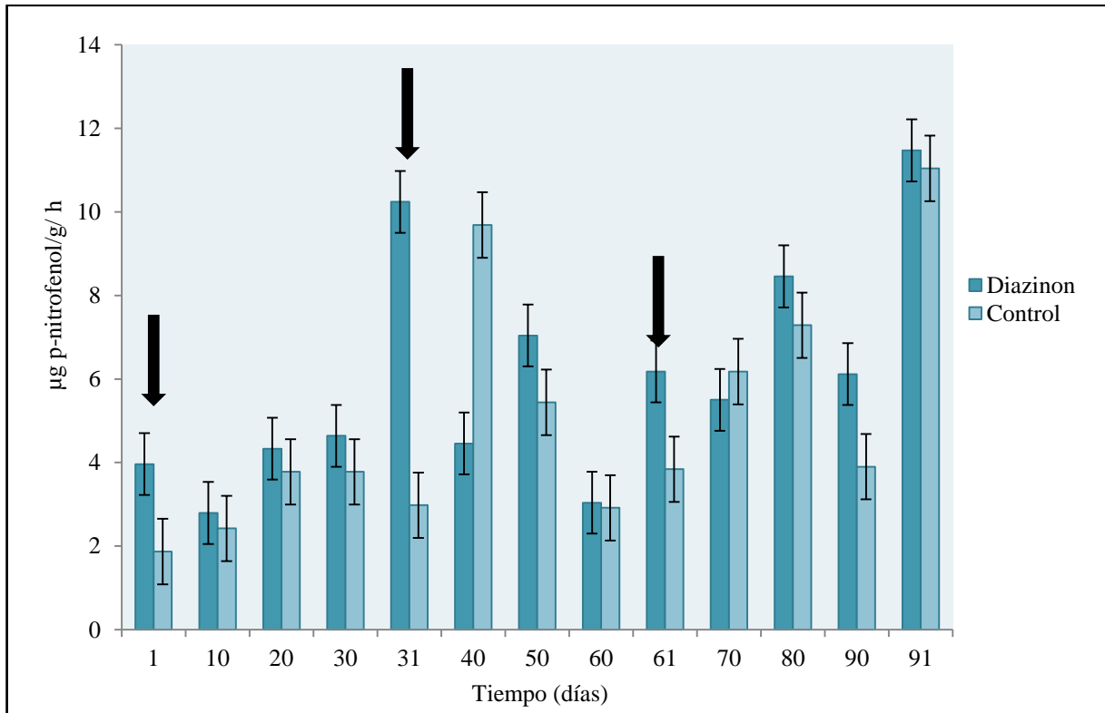
Figura 6. Efecto de 3 aplicaciones sucesivas de diazinón ( 40 \text{ mg ia kg}^{-1} ) sobre la actividad fosfatasa ácida. Las flechas indican el tiempo de aplicación.
