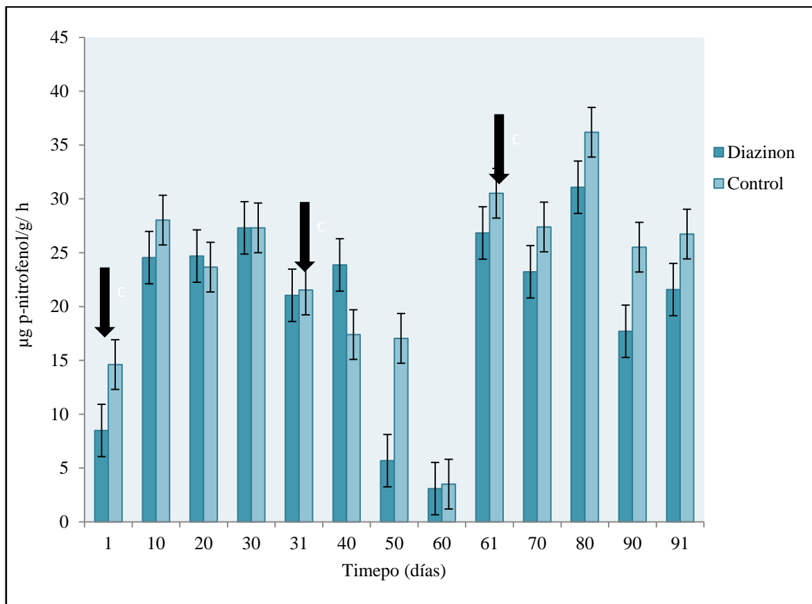
Figura 7. Efecto de 3 aplicaciones sucesivas de diazinón ( 40 \text{ mg ia kg}^{-1} ) sobre la actividad fosfatasa alcalina. Las flechas indican el tiempo de aplicación.
