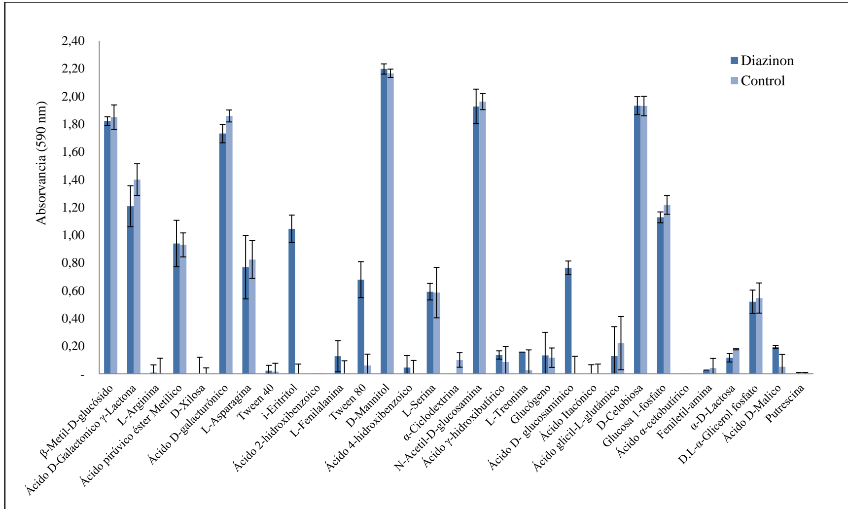
Figura 14. Perfil del nivel fisiológico de la comunidad microbiana (CLPP) al día 10 de evaluación.
